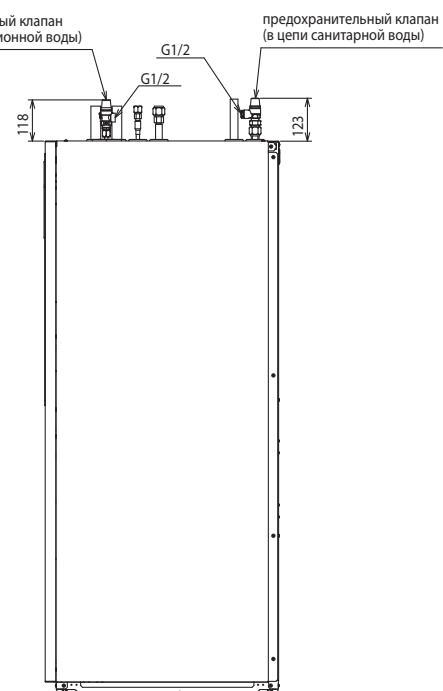
Вид справа
