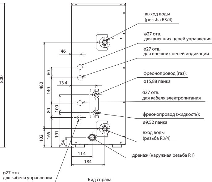
Вид справа
