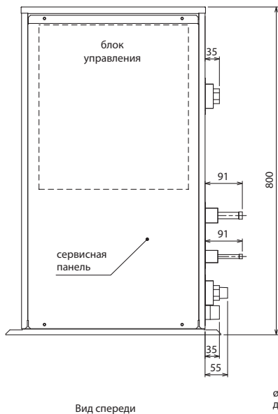
Вид спереди
